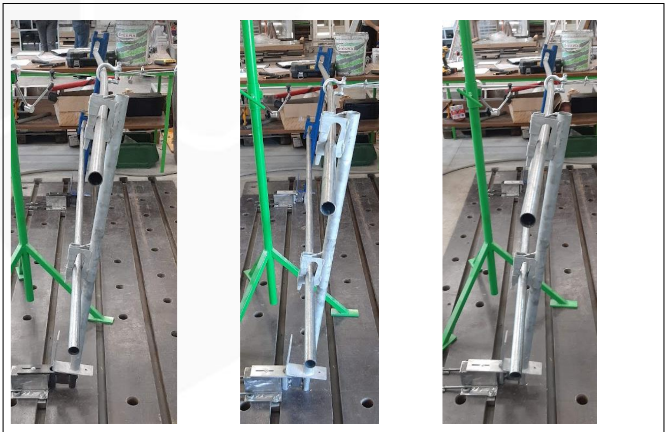
Garde-corps sollicité par la charge r_{U,i}^a
